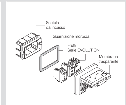
Versione da incasso - IP55.
