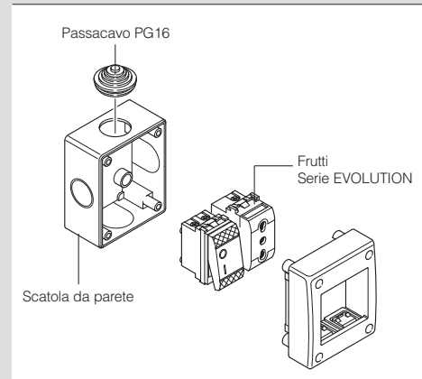
Versione da parete - IP40.
