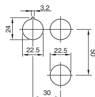
Hole EN 60947-5-1
